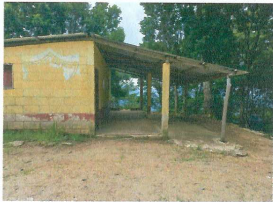
Foto 3: Cambio de pilares, estructura de techo madera a metal y cubierta de lámina troquelada calibre 26 del corredor
